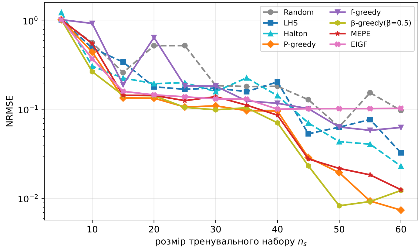
Збіжність помилки сурогата для f
